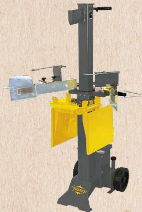
CJEPAČ ZA DRVA 7T 230V 3000W ADK* 752689
